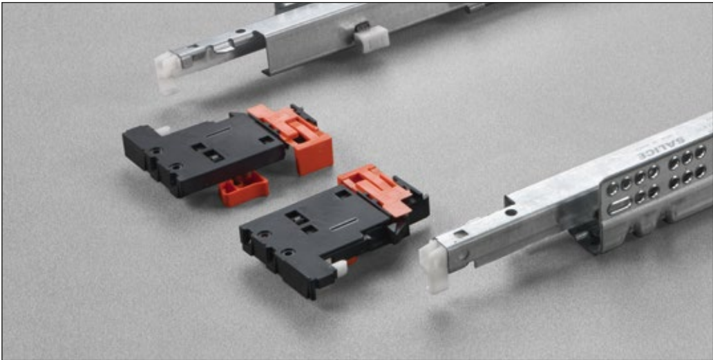
Detail des Clips mit 3 integrierten werkzeuglosen Verstellungen (Höhen-, Tiefen-, und Seitenverstellung).
